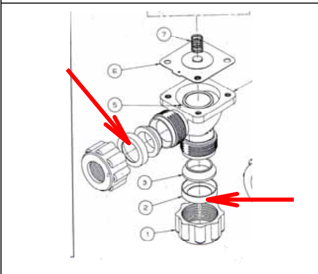
图 5. 所有 DD 型脉冲阀，配有铁环
