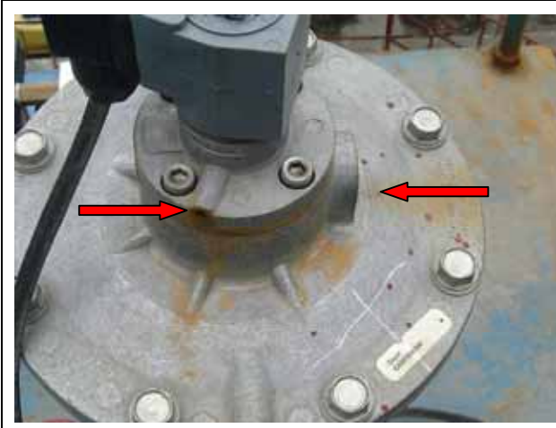
图 1. 气体内含有铁锈和杂物，堵塞出气孔
