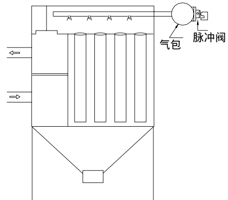
图 12. 对气箱喷吹时，喷吹管的两侧均匀地开直径为 30 mm 的喷吹孔，对压缩空气进行导流。请向深圳沃尔士公司索取示意图。
