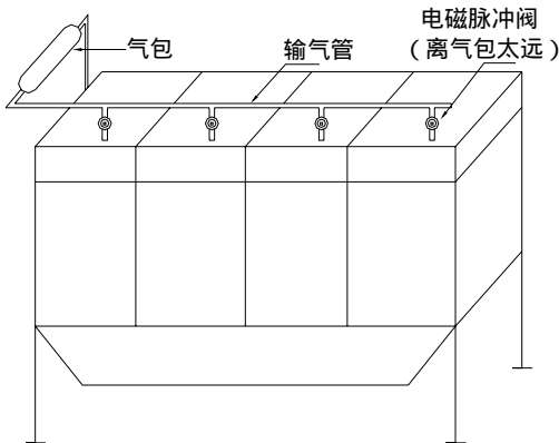
图 9. 在传统的气箱清灰系统中，脉冲阀离气包太远，造成喷吹后阀门进气管呈负压，引起“共鸣现象”。
